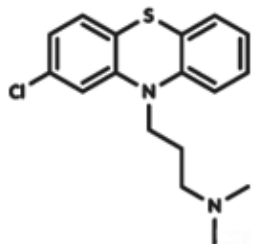
Molécula da clorpromazina
