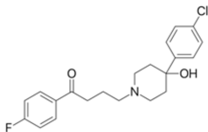
Molécula do haloperidol
