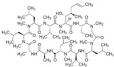
Estrutura da molécula de ciclosporina
