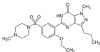
Molécula do sildenafil
